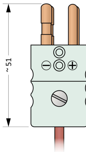
Obrázek 12U.7: MTCK-4S
