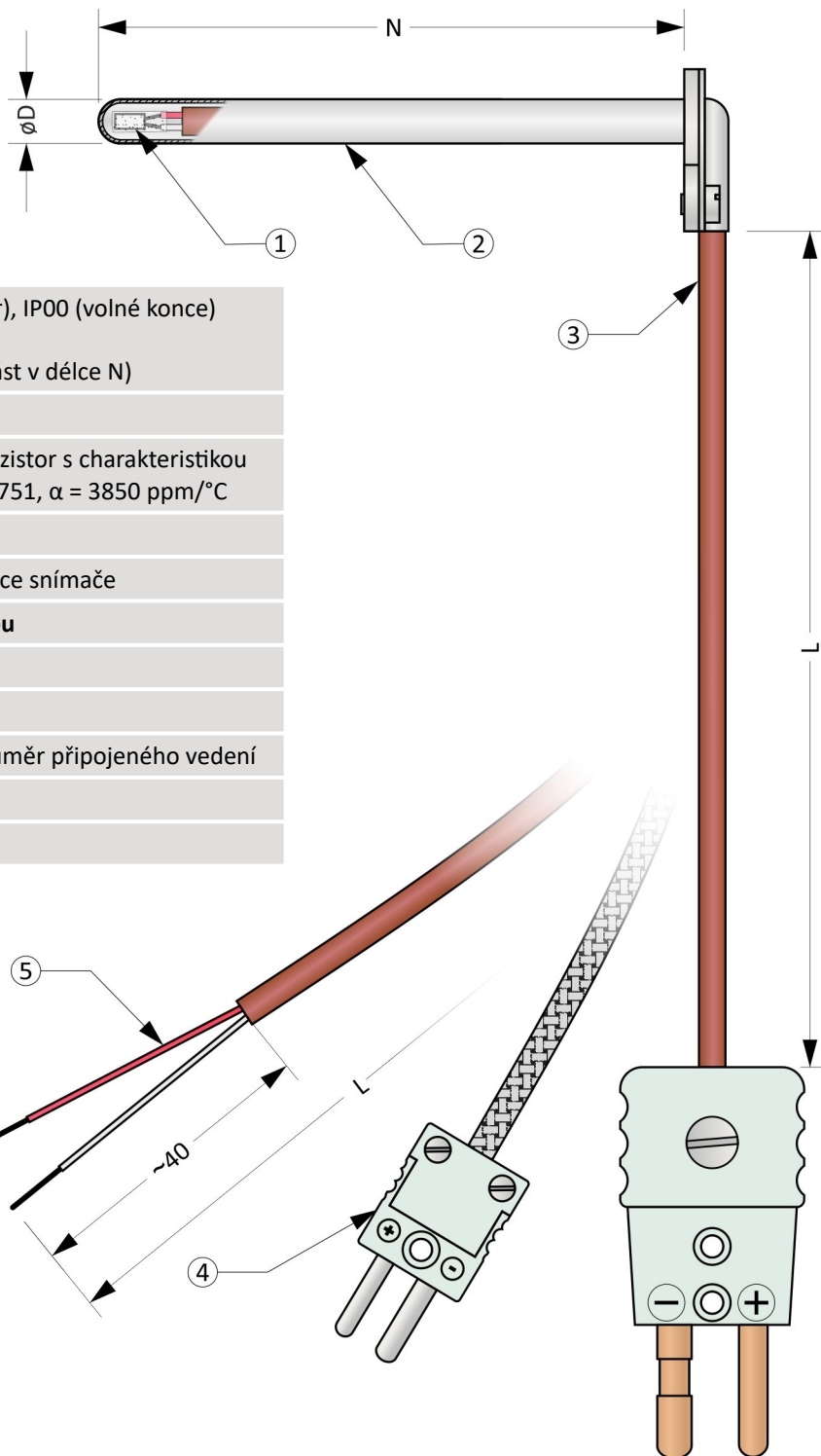
Obrázek 12U.1: MTR12U
