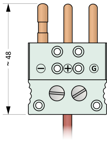
Obrázek 12U.6: MTCK-3S
