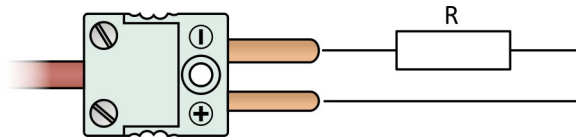
Obrázek 11.18: RTD v dvou vodičovém zapojení s miniaturním konektorem
